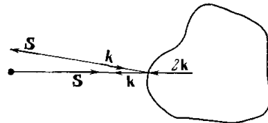
Рис. 6. Отражение луча, распространяющегося в среде с \epsilon < 0 и \mu < 0 от идеально отражающего тела.
