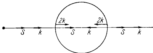
Рис. 8. Прохождение луча через шар с \epsilon < 0 и \mu < 0 , падающий в вакууме. Черной точкой обозначен источник излучения.
