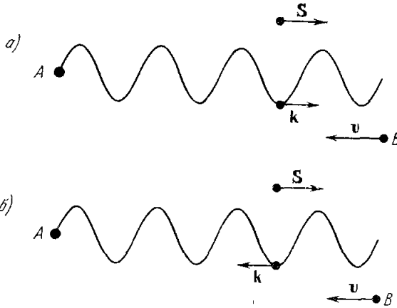
Рис. 1. а) Допплер-эффект в правом веществе. б) Допплер-эффект в левом веществе. Буквой А обозначен источник излучения, буквой В — присмник.
