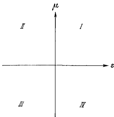
Рис. 7. Диаграмма \varepsilon - \mu .
