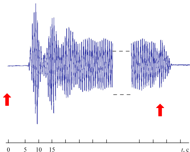
Рис. 1. Химически индуцированное радиочастотное излучение протонов, испускаемое молекулами хинона. Сигнал регистрируется на частоте 100 МГц; стрелки указывают моменты включения и выключения фотохимической накачки.
